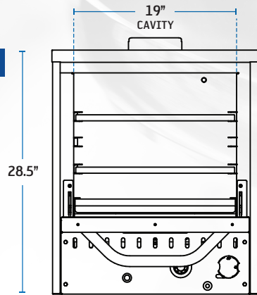
SRP0-24G
