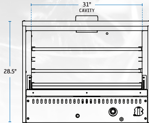
SRP0-36G
