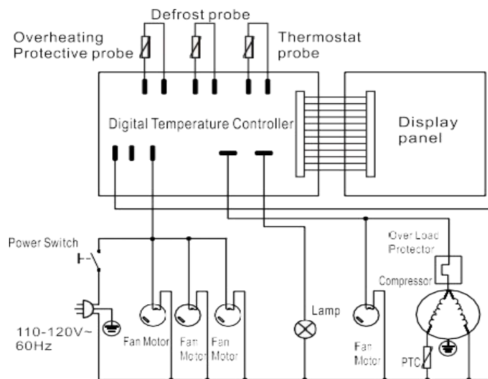
TMB36/TMB48
