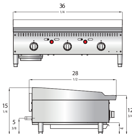
ATMG-36T
